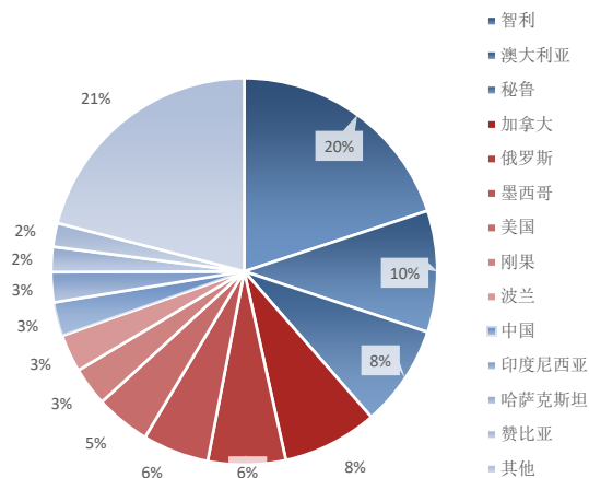
图 4：2021 年全球铜矿储量分布
