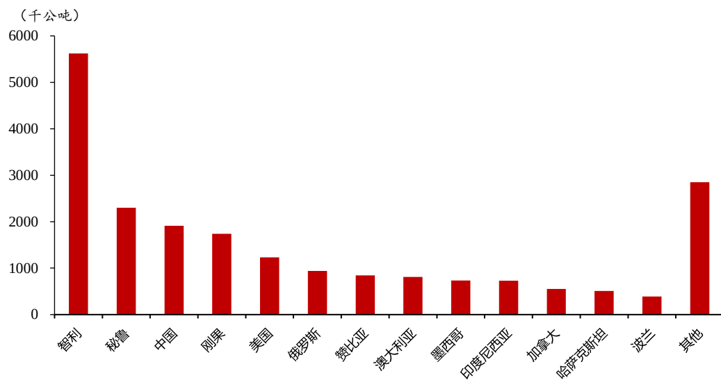
图 5：2021 年全球主要国家铜矿产量
