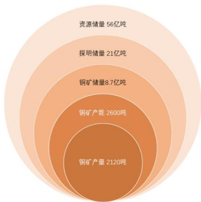
图3：2021 年全球铜矿产量与储量
